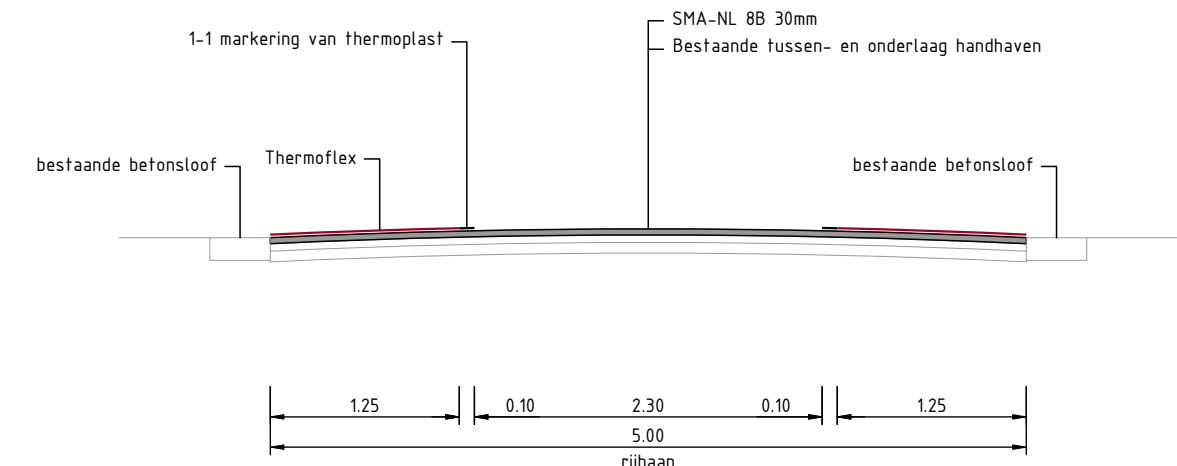
Dwarsprofiel C-C Schaal 1 : 50
