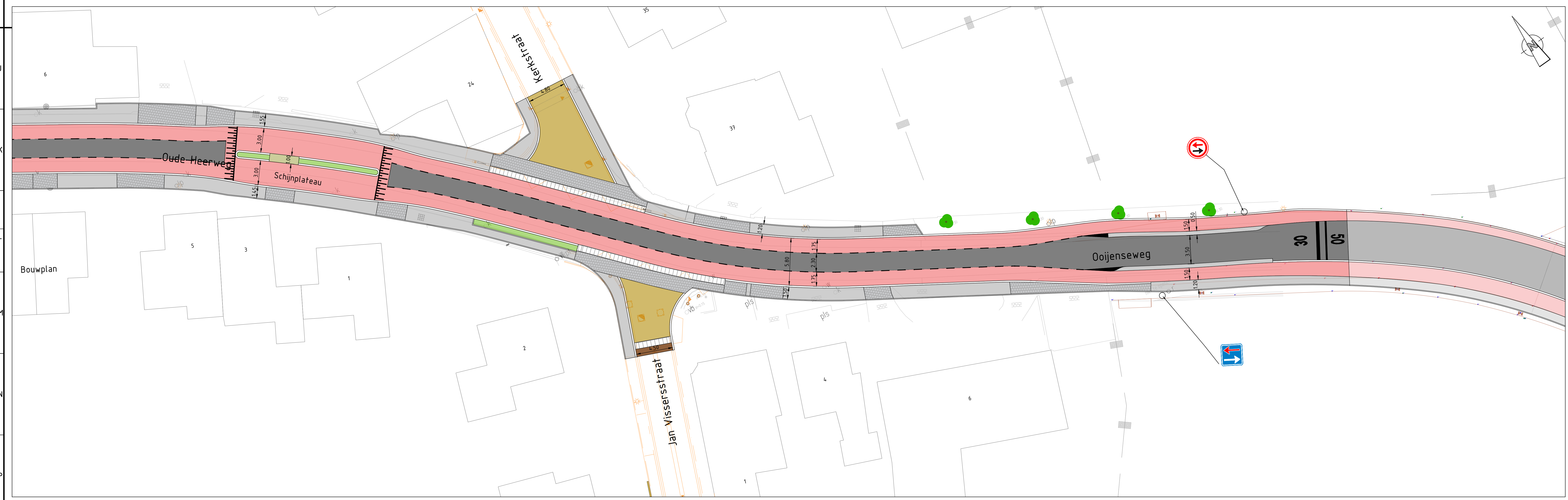
Overzicht 5 SCHAAL 1:200
